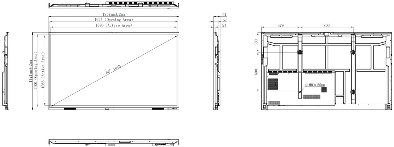
86": ST-86-CONNECT-PRO5
